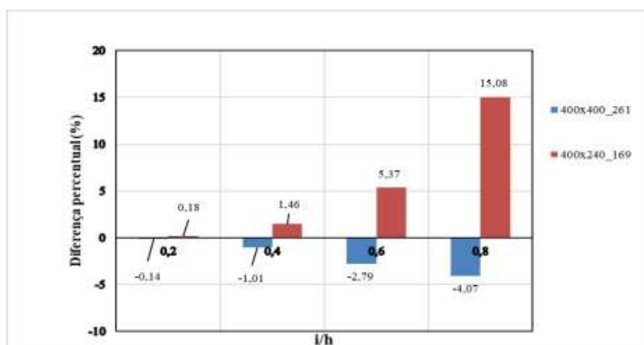
Figura 4: Efeito da relação i/h nos deslocamentos verticais, no central dos painéis 400x400 e 400x240
